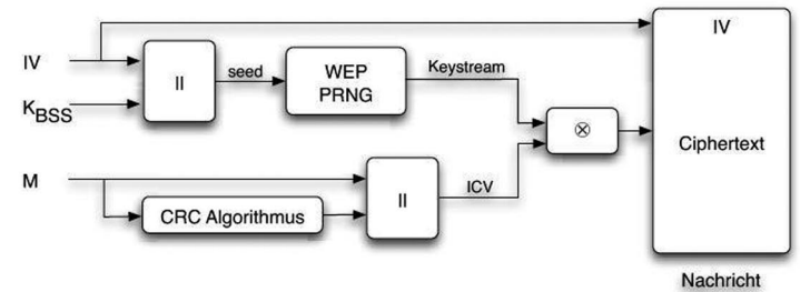
Abb. 26: WEP-Verschlüsselung
