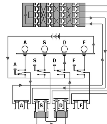
Abb. 35: Skizze: Prinzipieller Aufbau der Enigma aus Walzensatz, Lampenfeld, Tastatur und Steckerbrett
