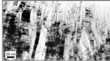
Abb. 36: Elektronenmikroskopische Aufnahme von Graphit-Basalebene im Querschnitt
