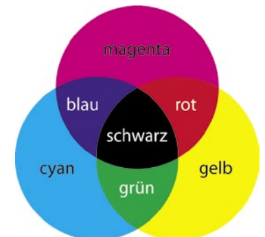
Abb. 45: Subtraktive Farbsynthese
