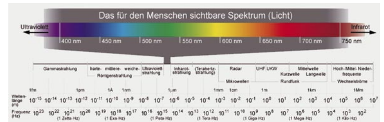
Abb. 43: Sichtbares Spektrum
