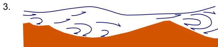
Dunes
