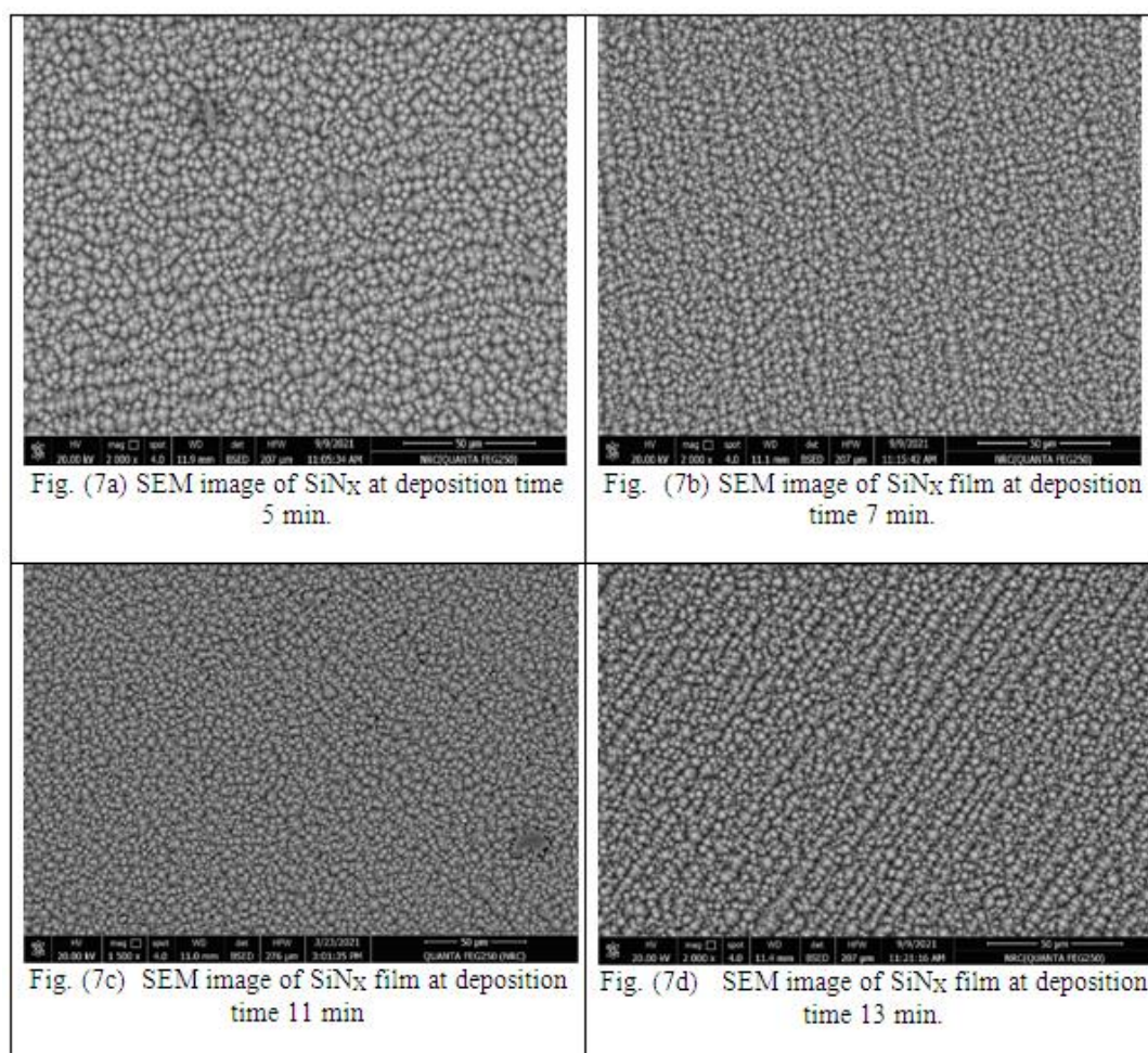
Fig.7. SEM images of solar cells for different SiN x film deposition times; (a) 5min., (b)7min., (c)11min.,(d)13min.
