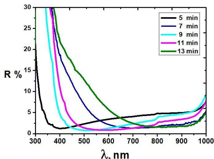
Fig.5. Reflectance of SiN x films at deposition times 5min., 7min., 9min., 11min., 13min.
