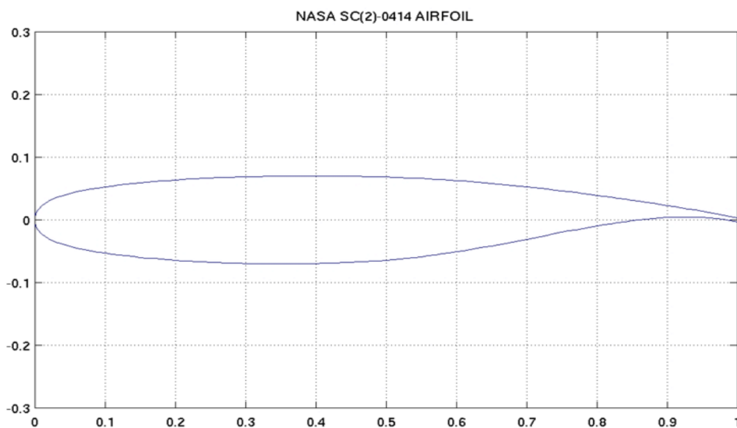
Fig.4: 0414 aero foil
