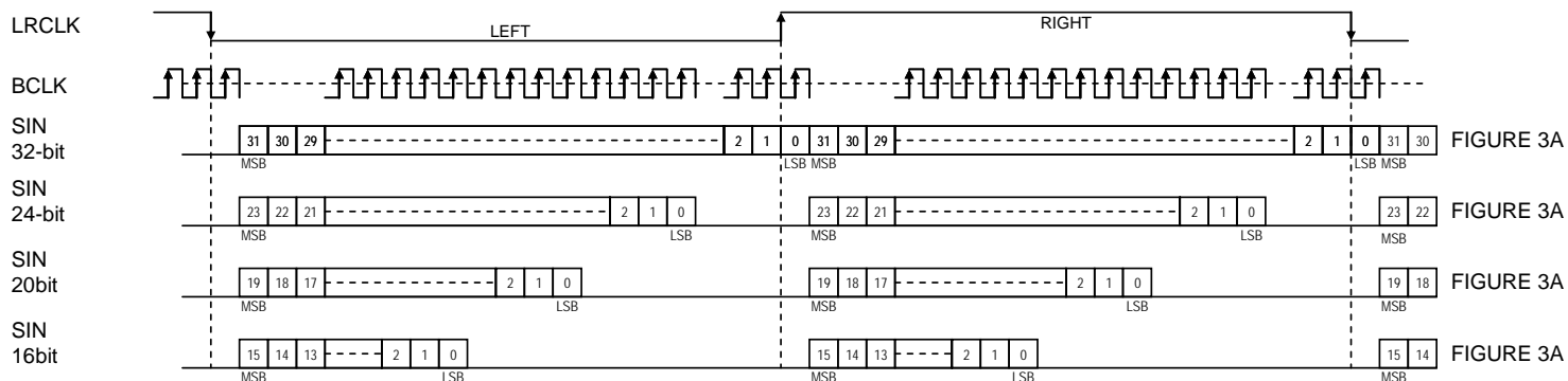
I2S FORMAT
