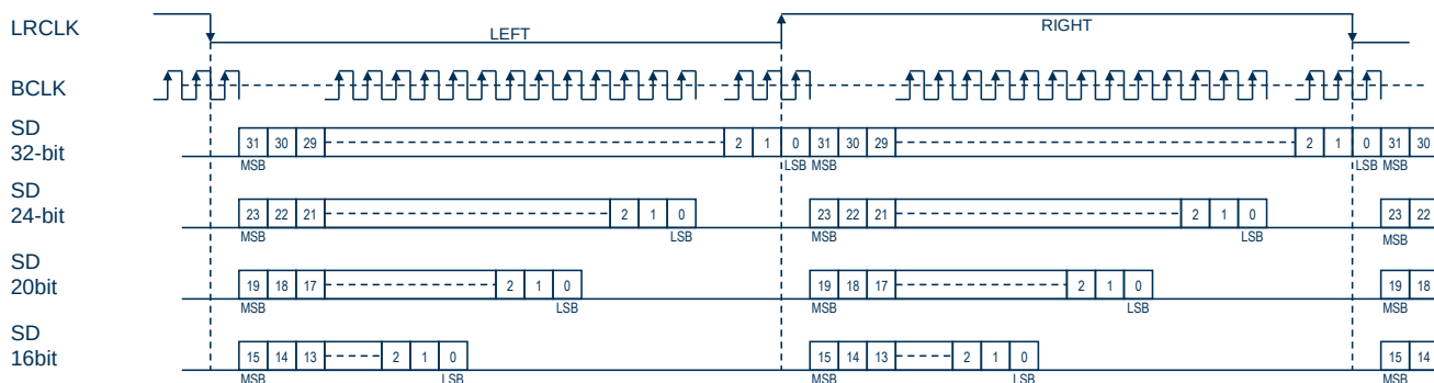
I2S FORMAT
