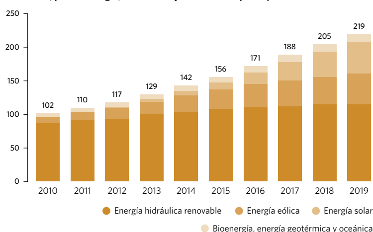
Capacidad de generación de energía eléctrica renovable instalada en los países en desarrollo, por tecnología, entre 2010 y 2019 (vatios per cápita)
