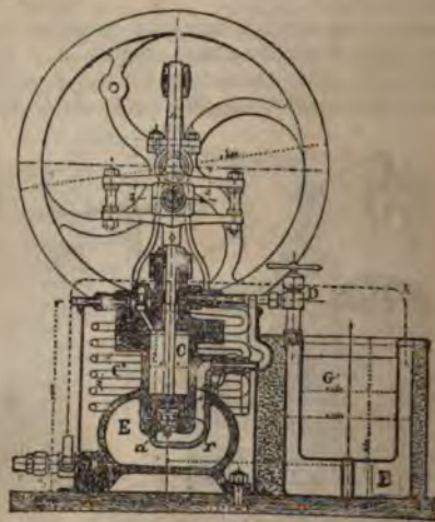
Фиг. 4. Машина с хлористым методом Венса (Vincent).
