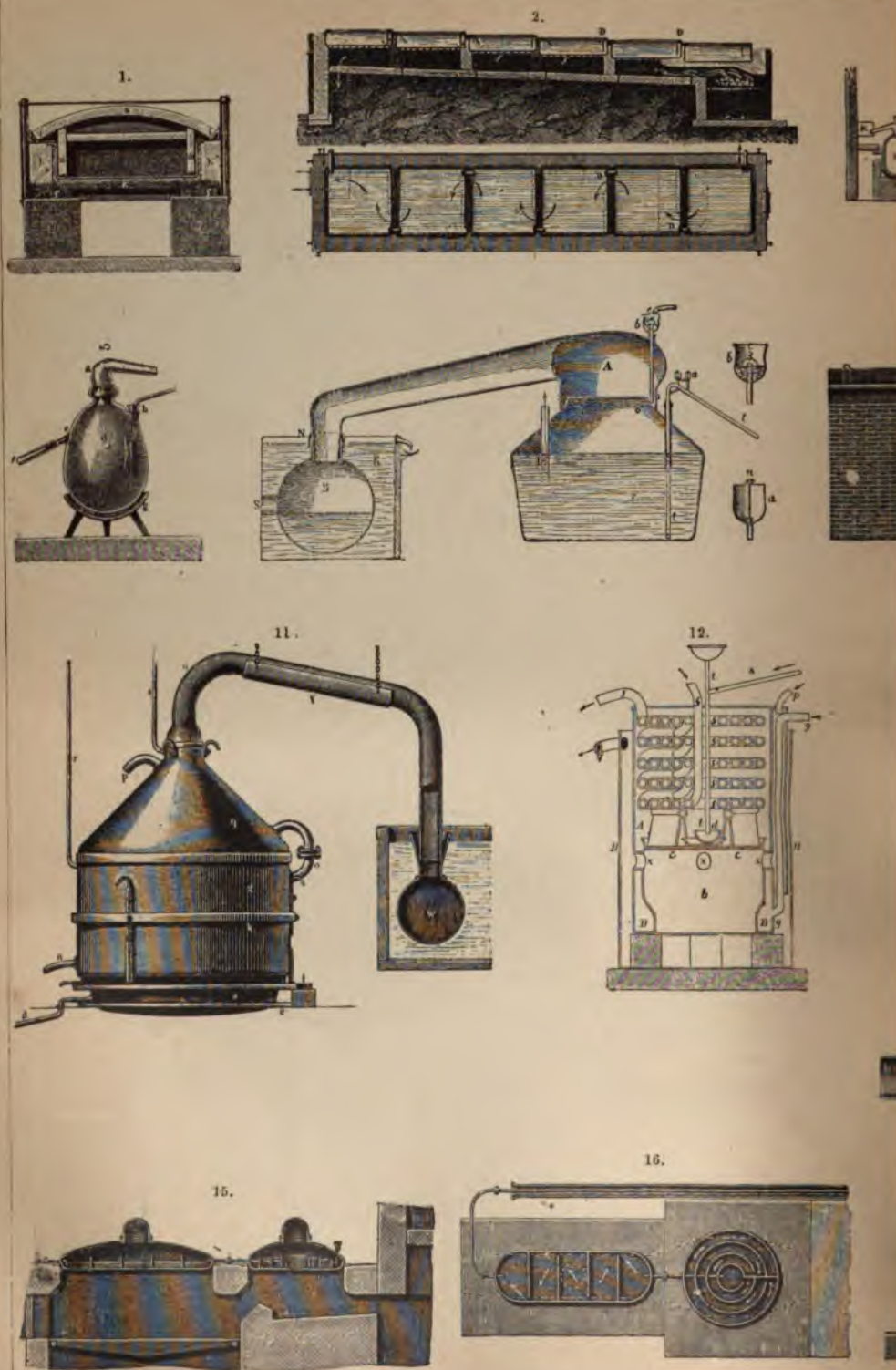
1. Стуже́ние до 60° В. съ ва́рьюномъ сверху (поперечный разръзъ). 2. То же съ ва́рьюномъ снизу (продольный разръзъ). 3. Стуже́ние до 60° В. въ стёклянныхъ ретортахъ. 4. Часть ретортнаго ота́жася въ пла́нъ. 5. Стёкляная реторта для Либиха (разръзъ). 6. Плоский платиновый кубъ Desmoutis, Lemaire & Co. 7 и 8. Кубъ системы Grenice (видъ сверху и снизу). 9 и 10. Кубъ системы Grenice (видъ сверху и снизу). 11 и 12. Стуже́ние по способу А. Кесслера въ Касермонь-Ферранъ (продольный и поперечный разръзъ).
