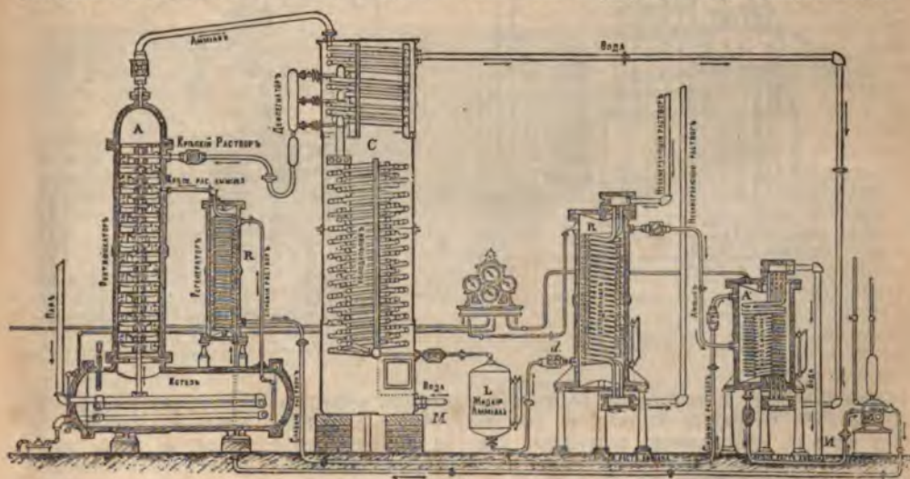
Фиг. 2. Абсорбционная амміачная машина Понтифекса и Вуда. Система Карре.
