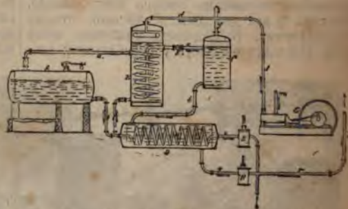
Фиг. 6. Способъ Линде для экономическаго полученія прозрачнаго льда изъ перегретой воды.
