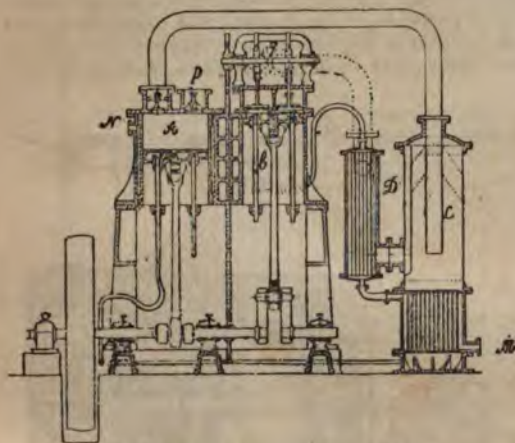
Фиг. 3. Воздушная машина С — ть Обера.
