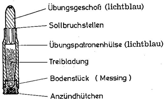
Aufbau einer Übungspatrone 7,62 mm x 51 DM18
