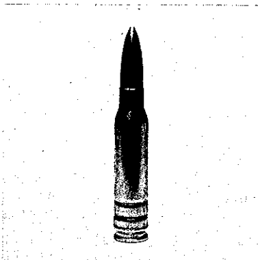
Exerzierpatrone 7,62 mm \times 51 DM20
