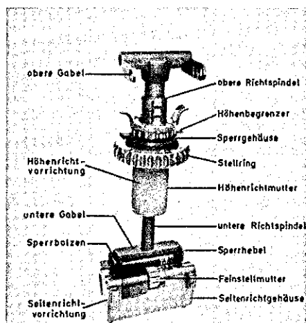
Richtvorrichtung
