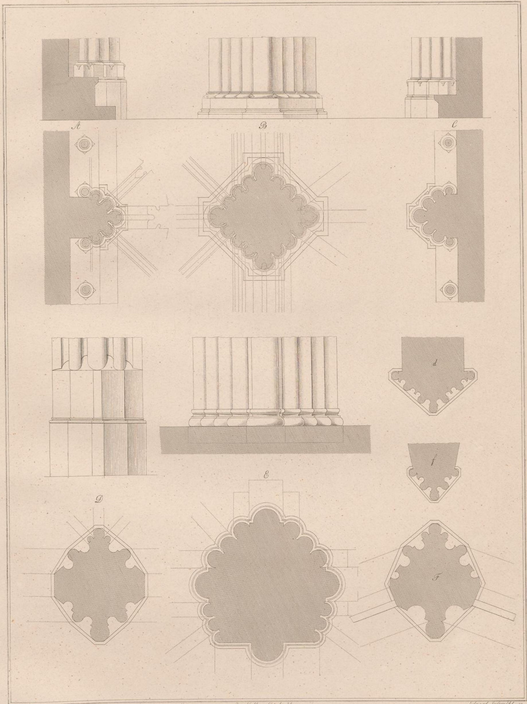
Détails des colonnes dans la Cathédrale à Fribourg.
