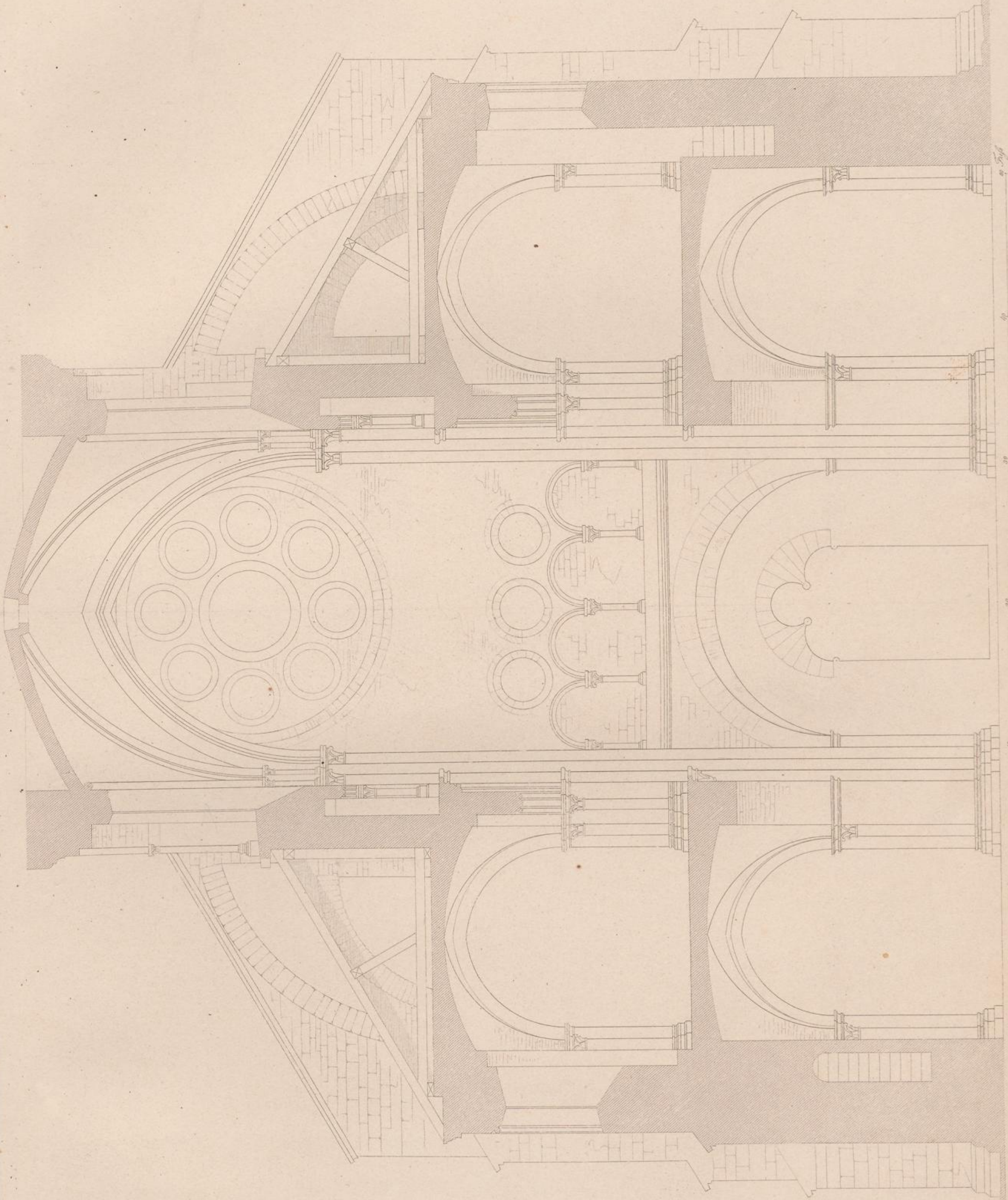
Coupe transversale
