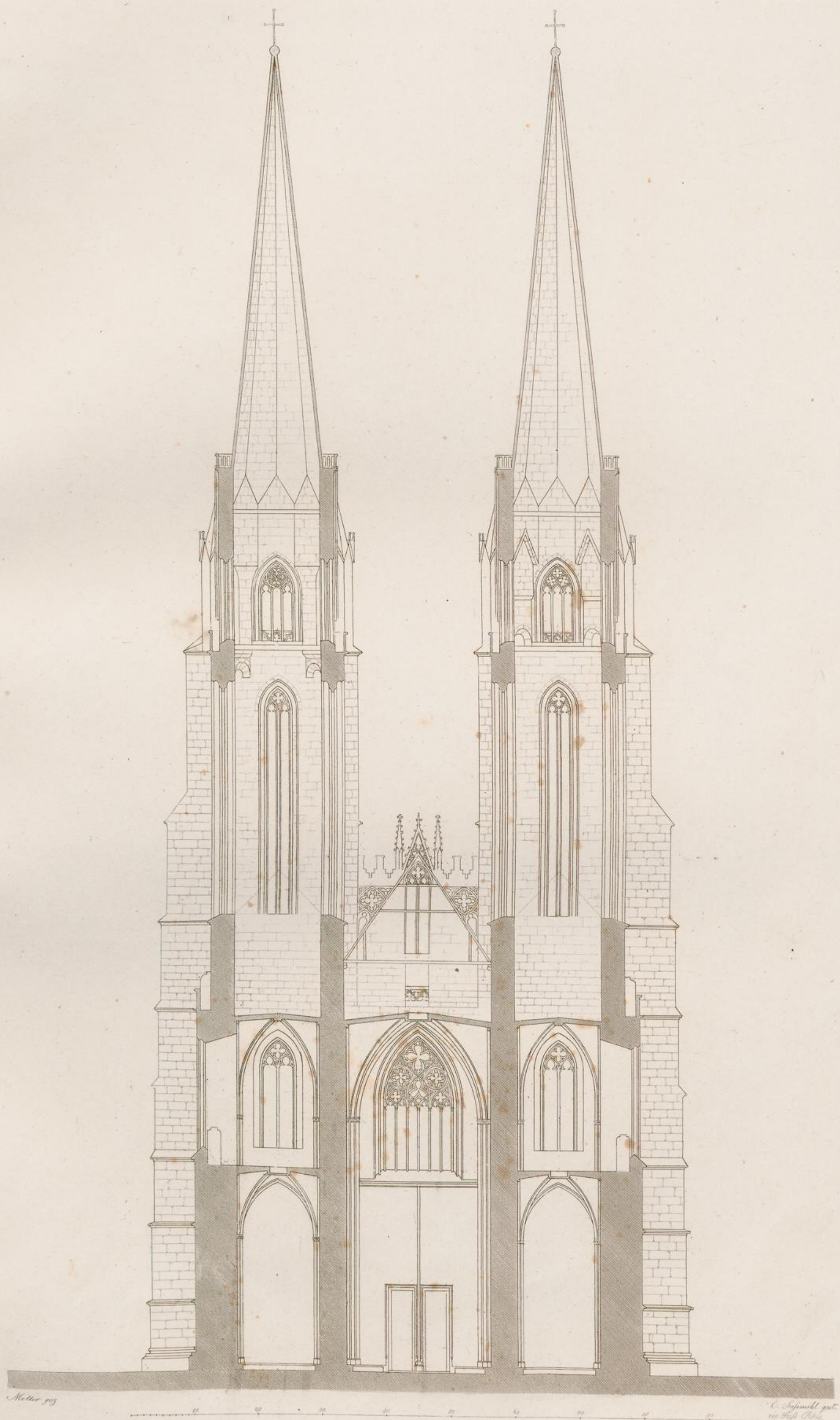
Durchschnitt der Thürme
