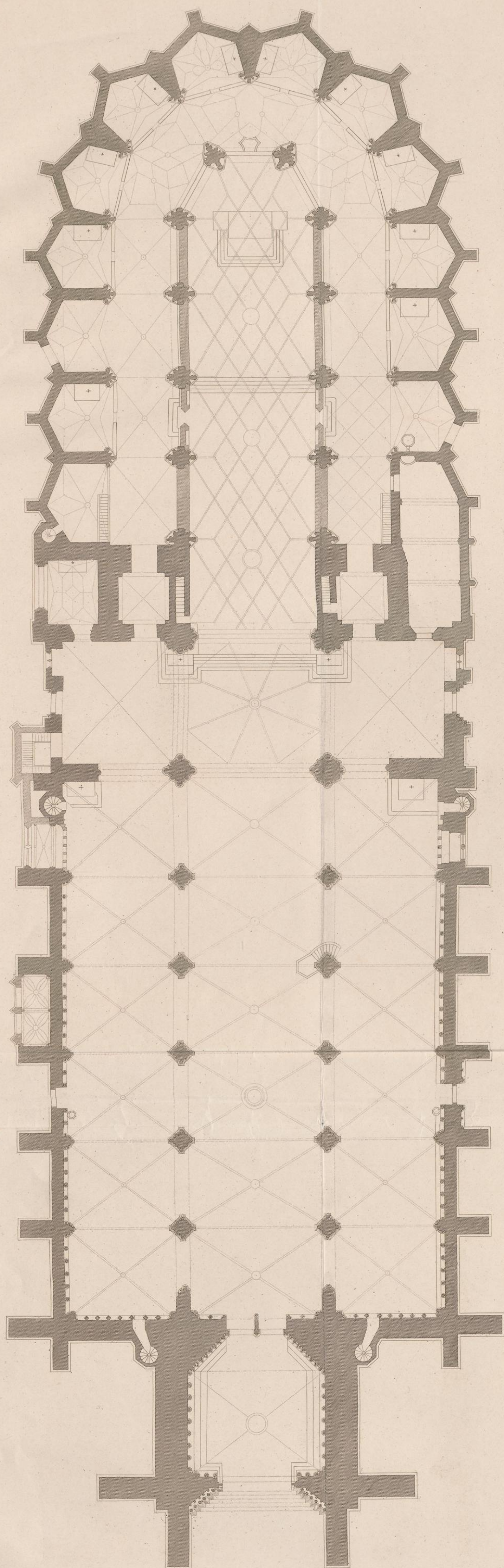
Grundriss der Kirche
