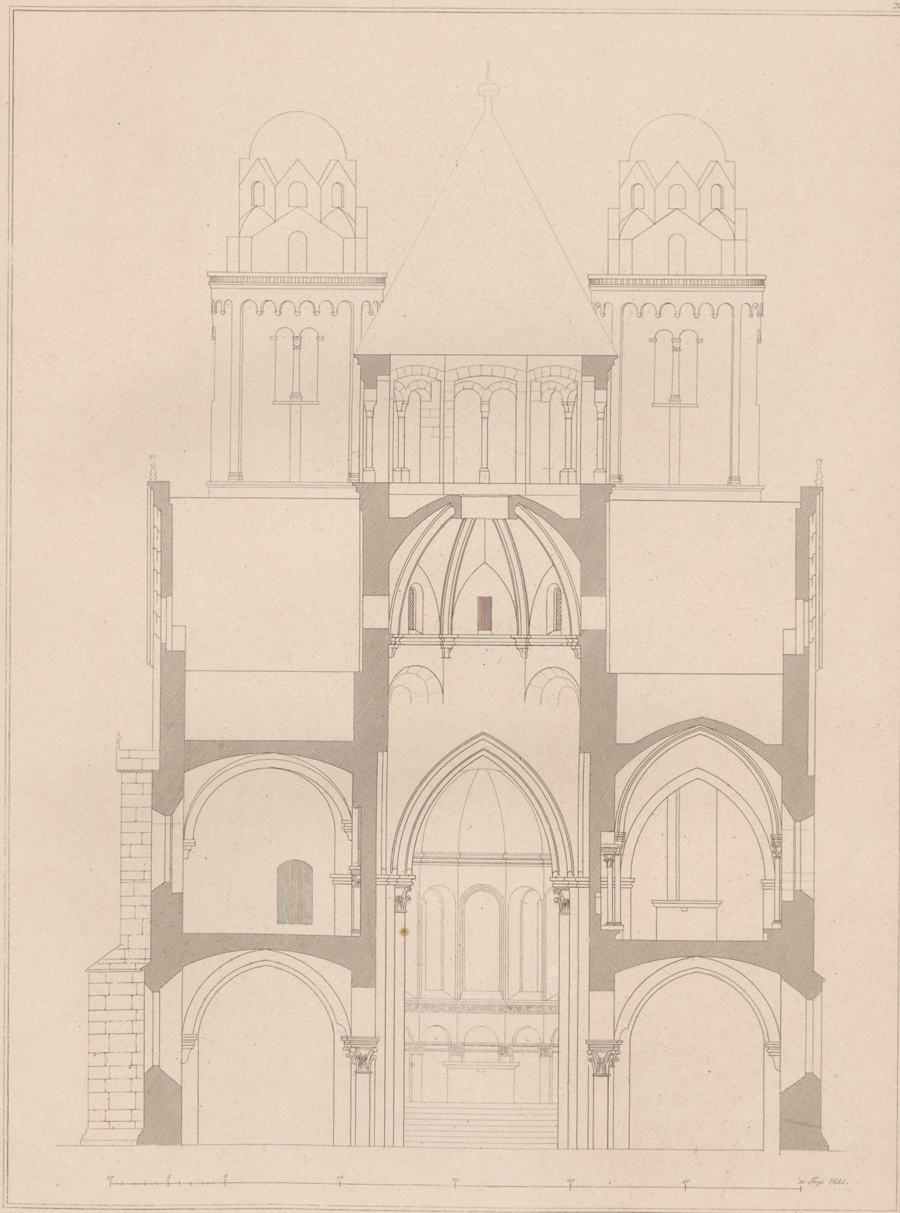
Durchschnitt der St. Paulskirche zu Worms.
