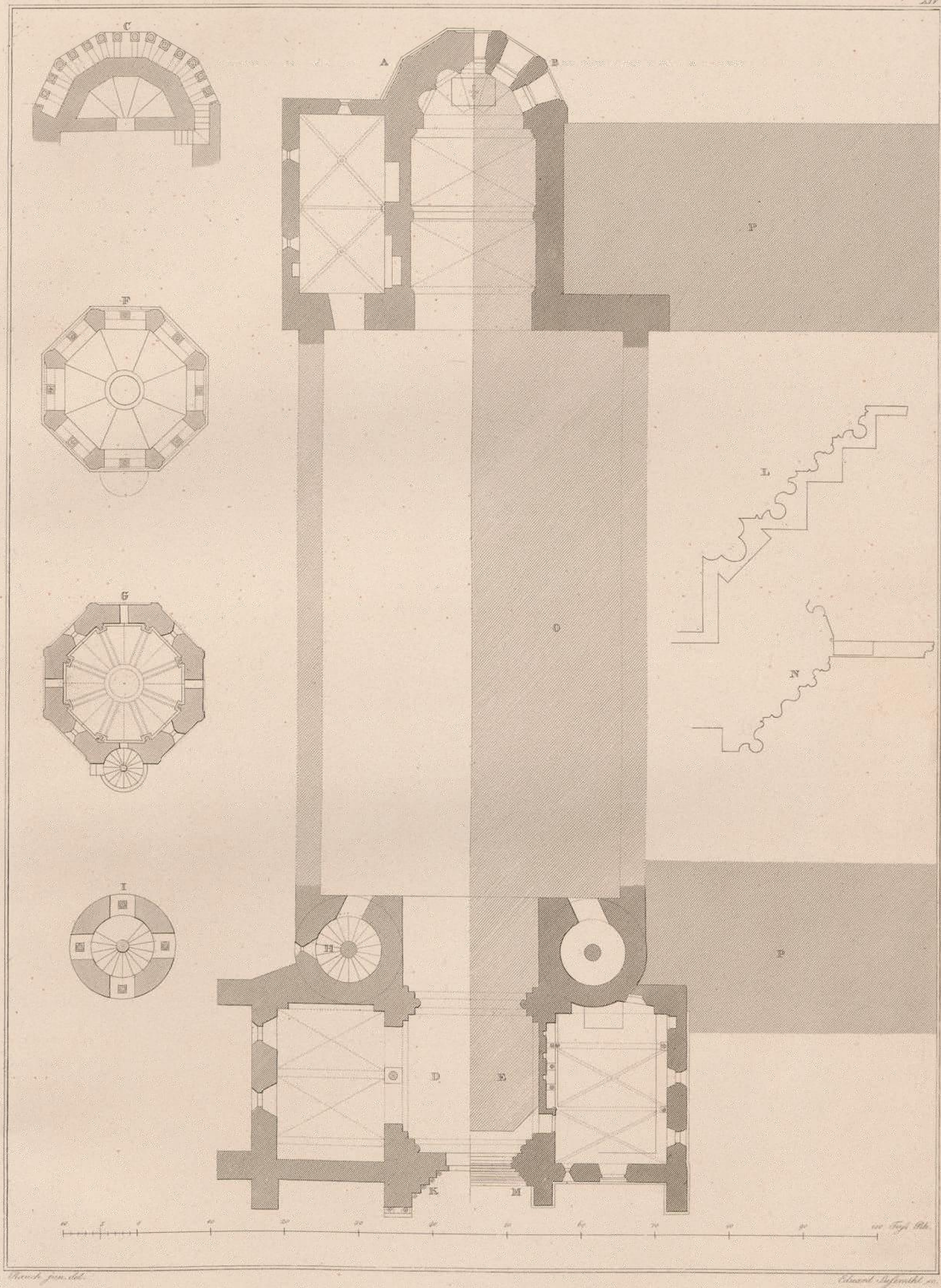
Grundriß der St. Paulskirche zu Worms
