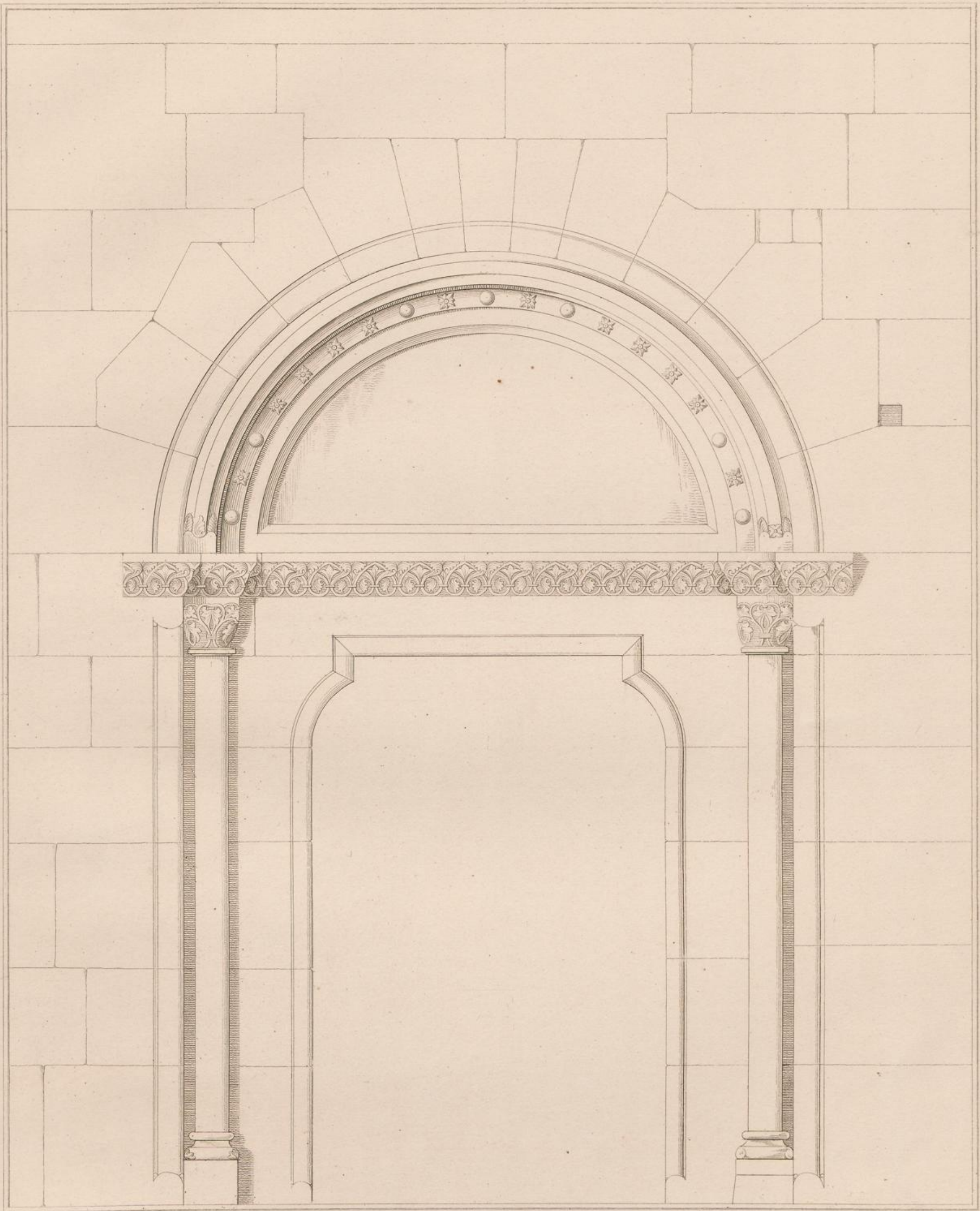
Nördliche Thüre am Münster zu Freiburg.
