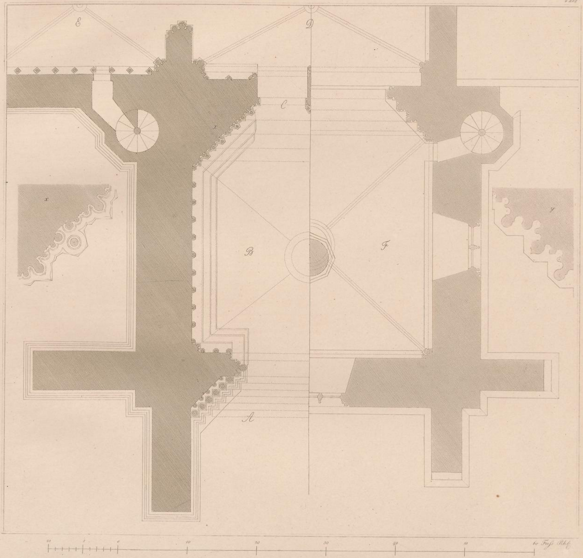
Grundriß des ersten und zweiten Stocks des Thurmes
