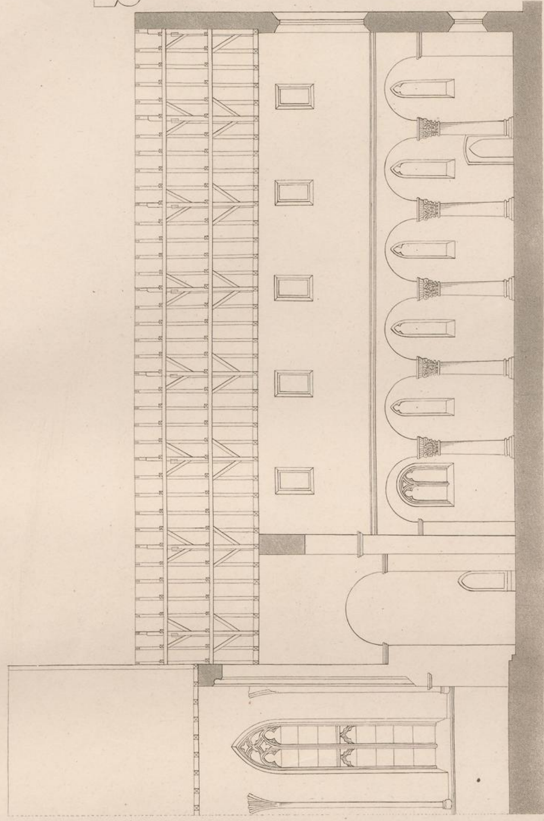
Längendurchschnitt.
