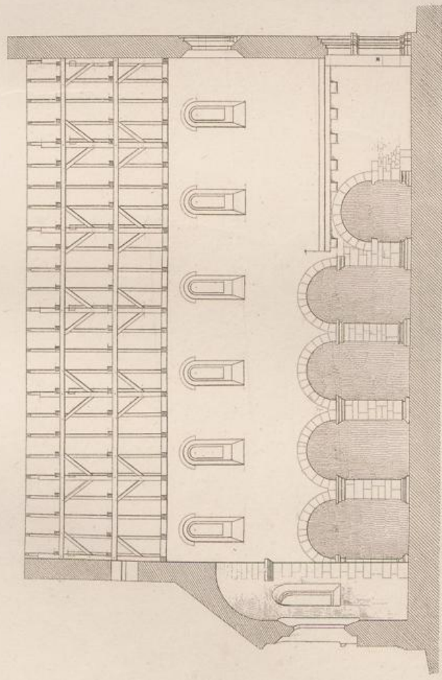
Längs-Durchschnitt
