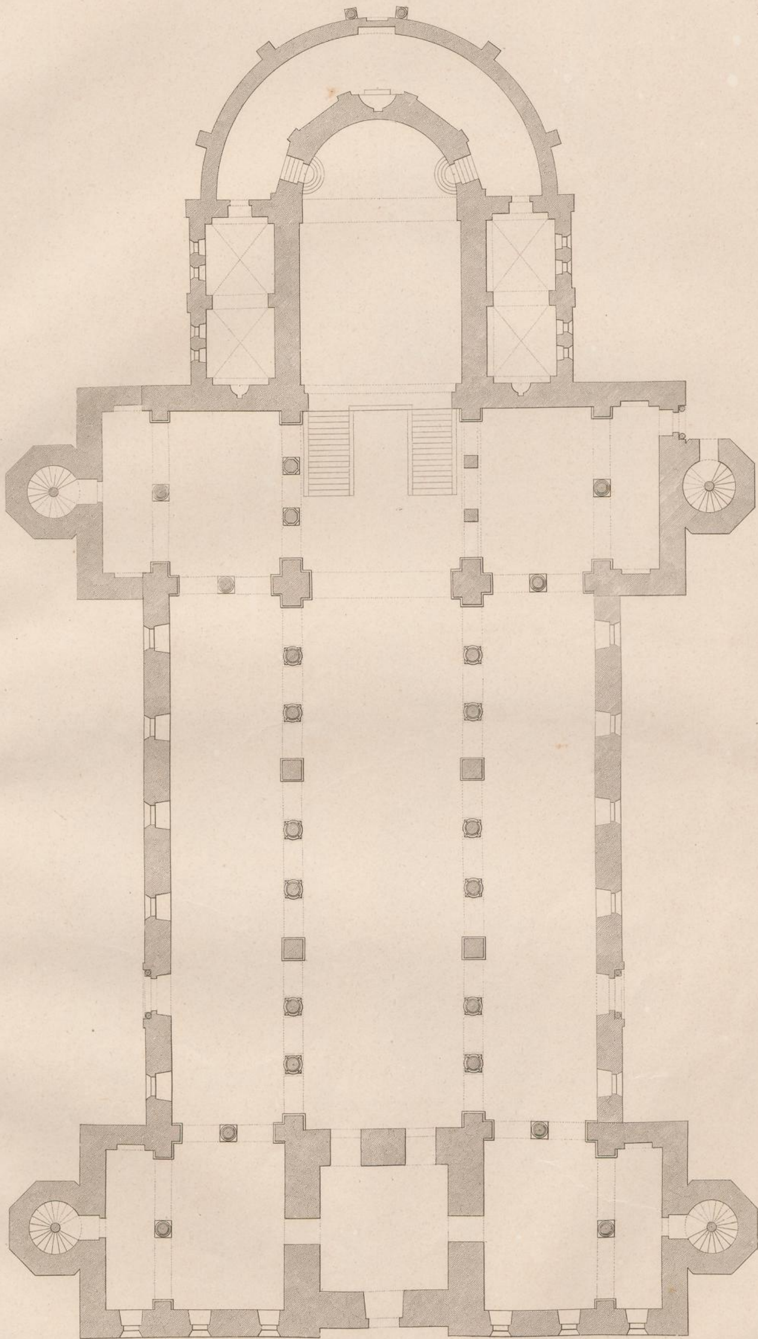
Grundriss der Kirche St. Michael zu Hildesheim.
