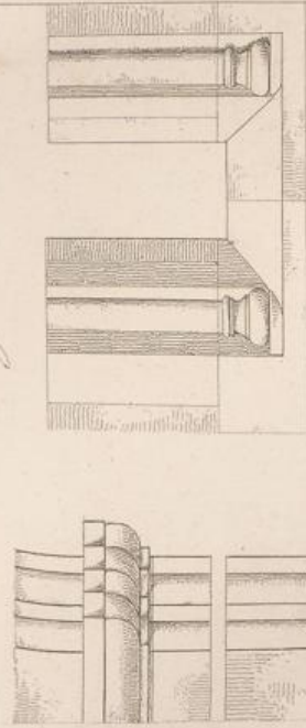
Ansicht und Grundriss der Fenster Details des Portals
