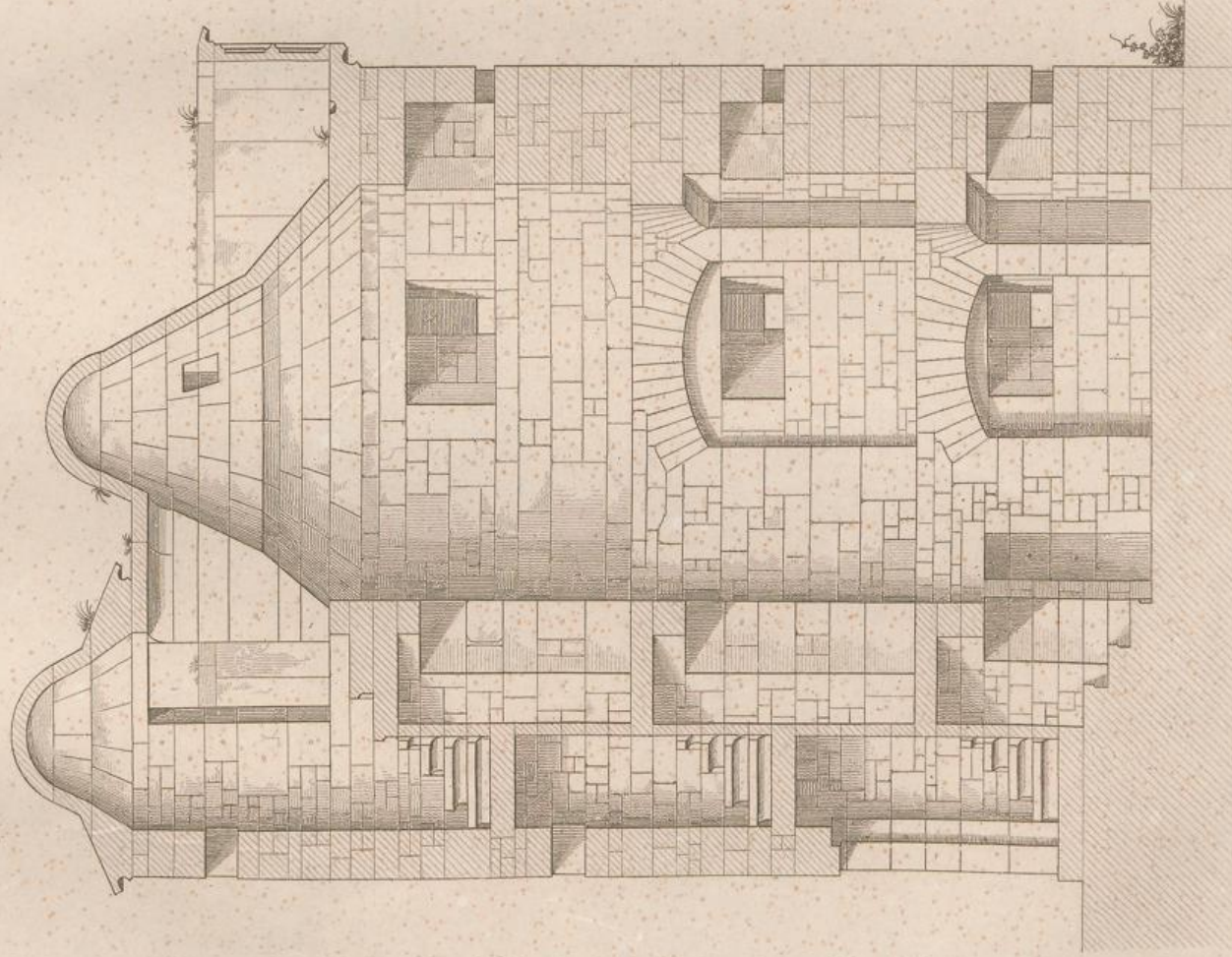
Querschnitt des südlichen Thurmes
