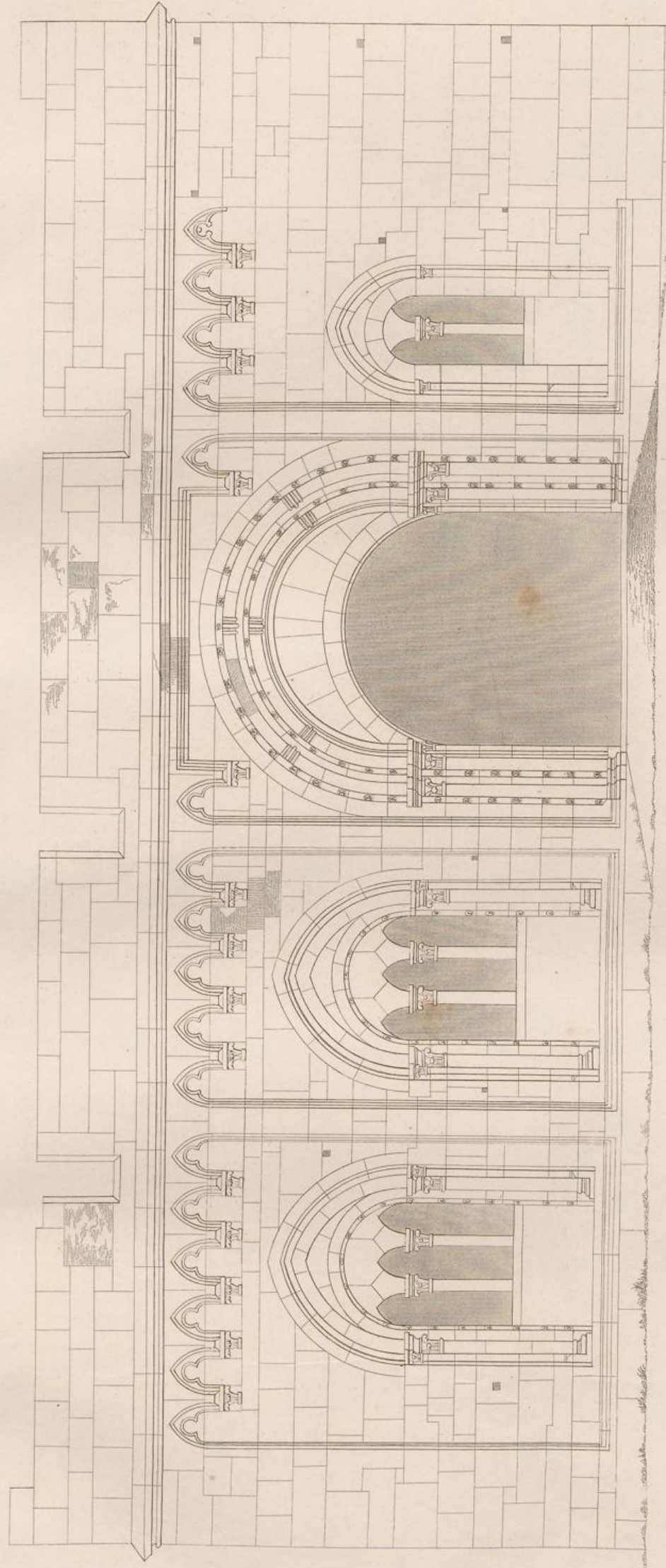
Vorhalle des Doms zu Freyburg
