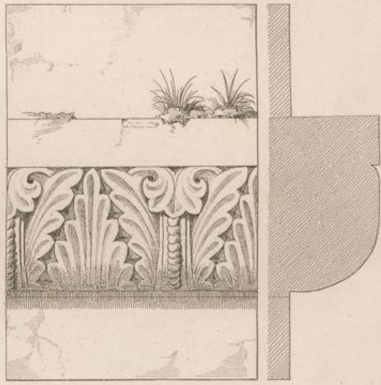
Kapitel der 2. Saculen im Inneren. Kämpfergesimse des Pallastes. Profil der Thorfahrt
