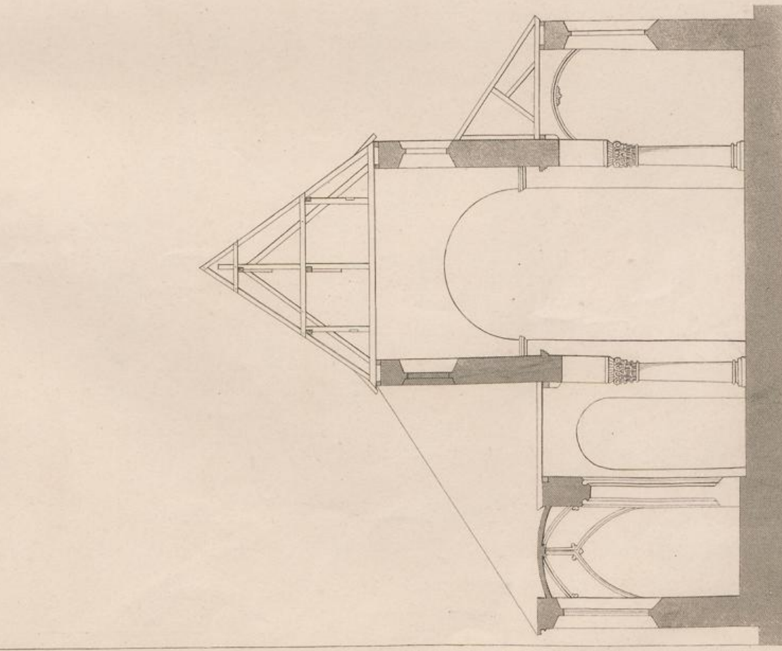
Querschnitt.
