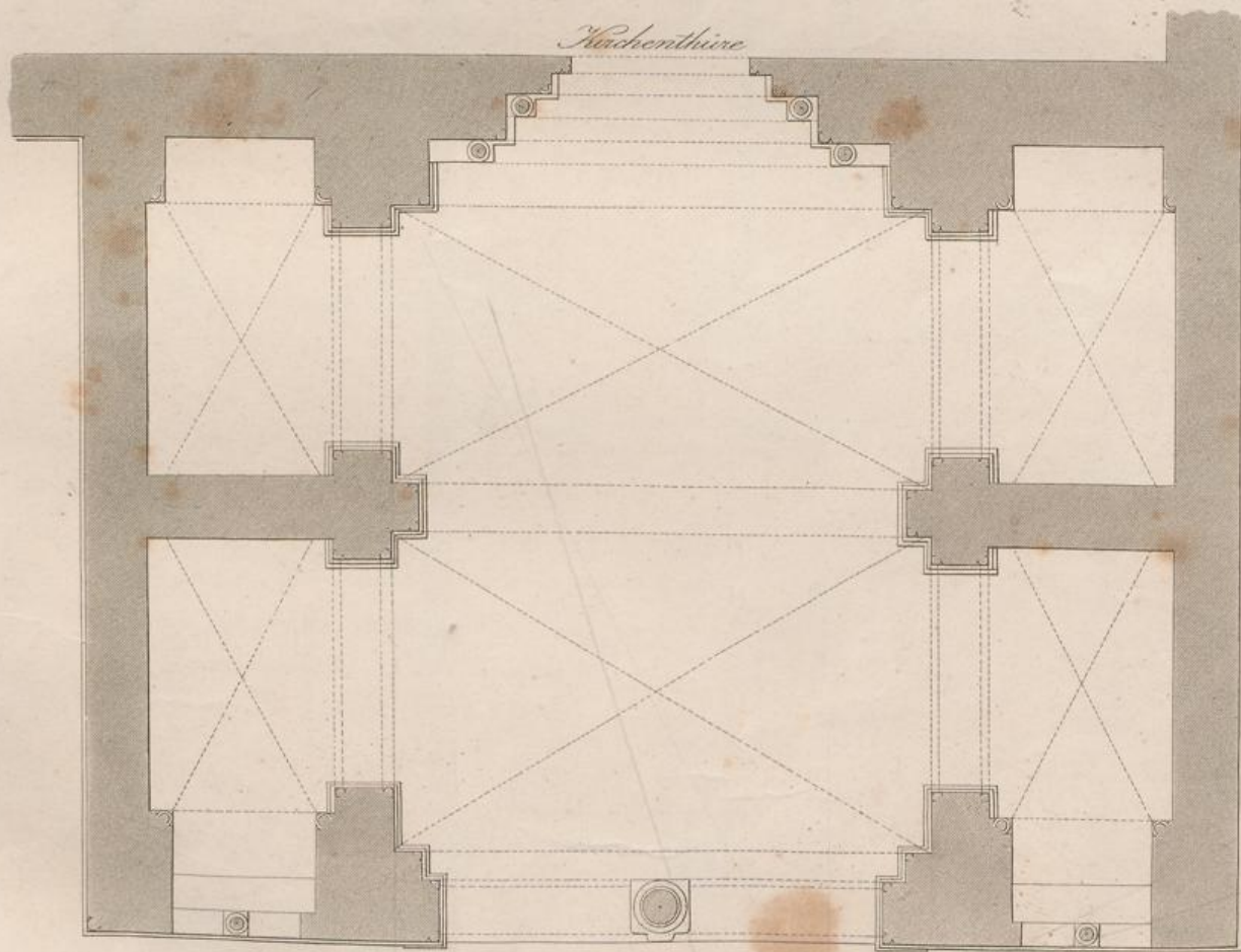
Grundriss
