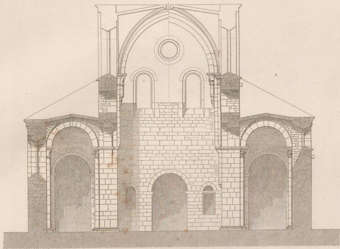
Querschnitt der Kirche
