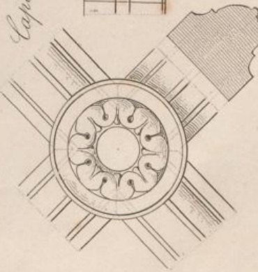
Schlufstein der Genölle.
