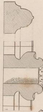
Schlufstein der Genölle.
