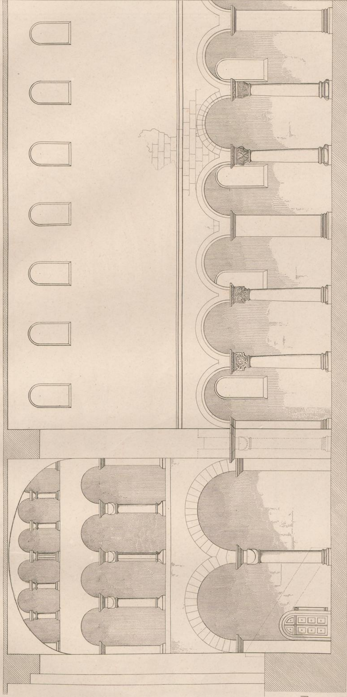
Längendurchschnitt
