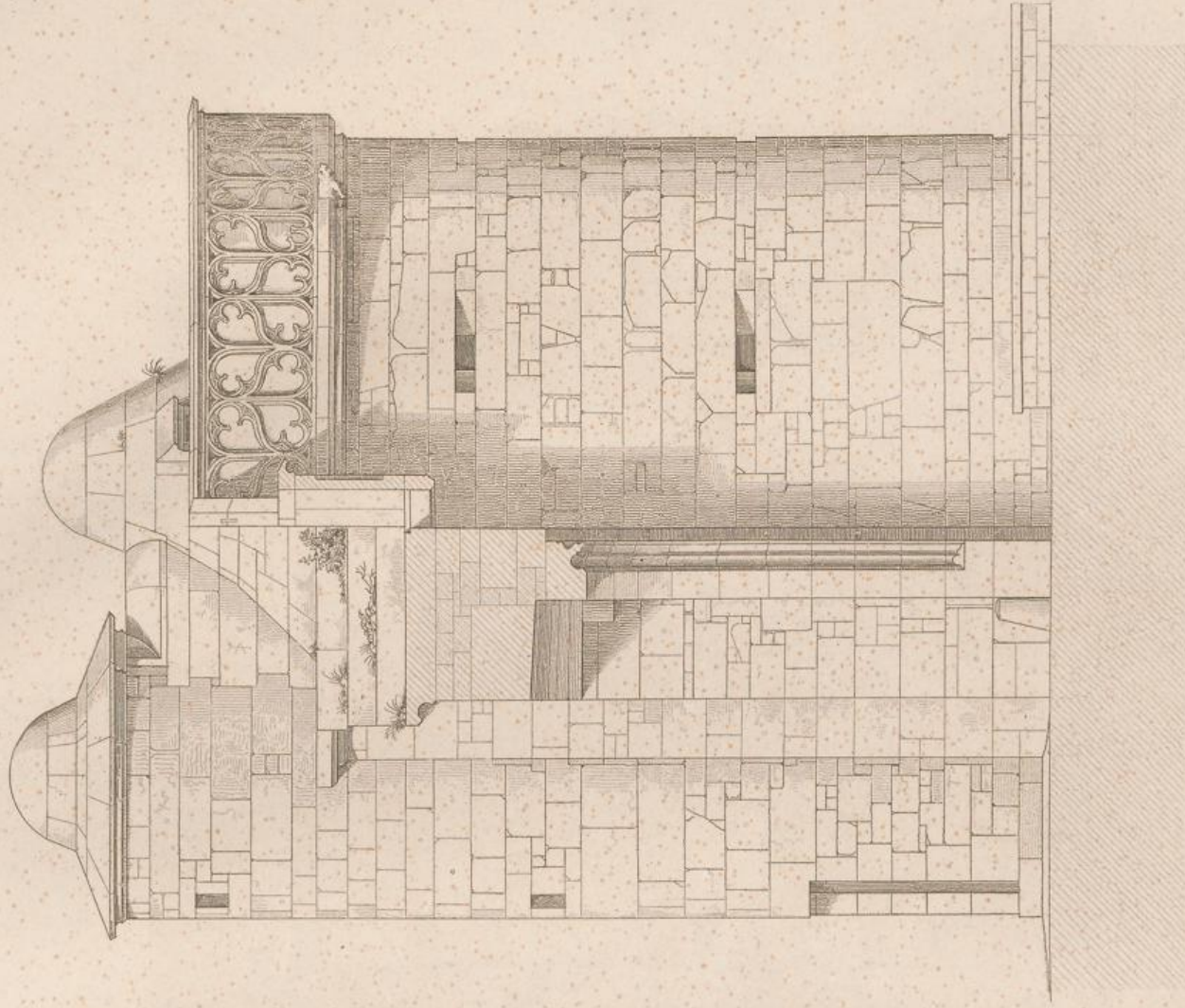
Querschnitt durch die Mitte des Thores
