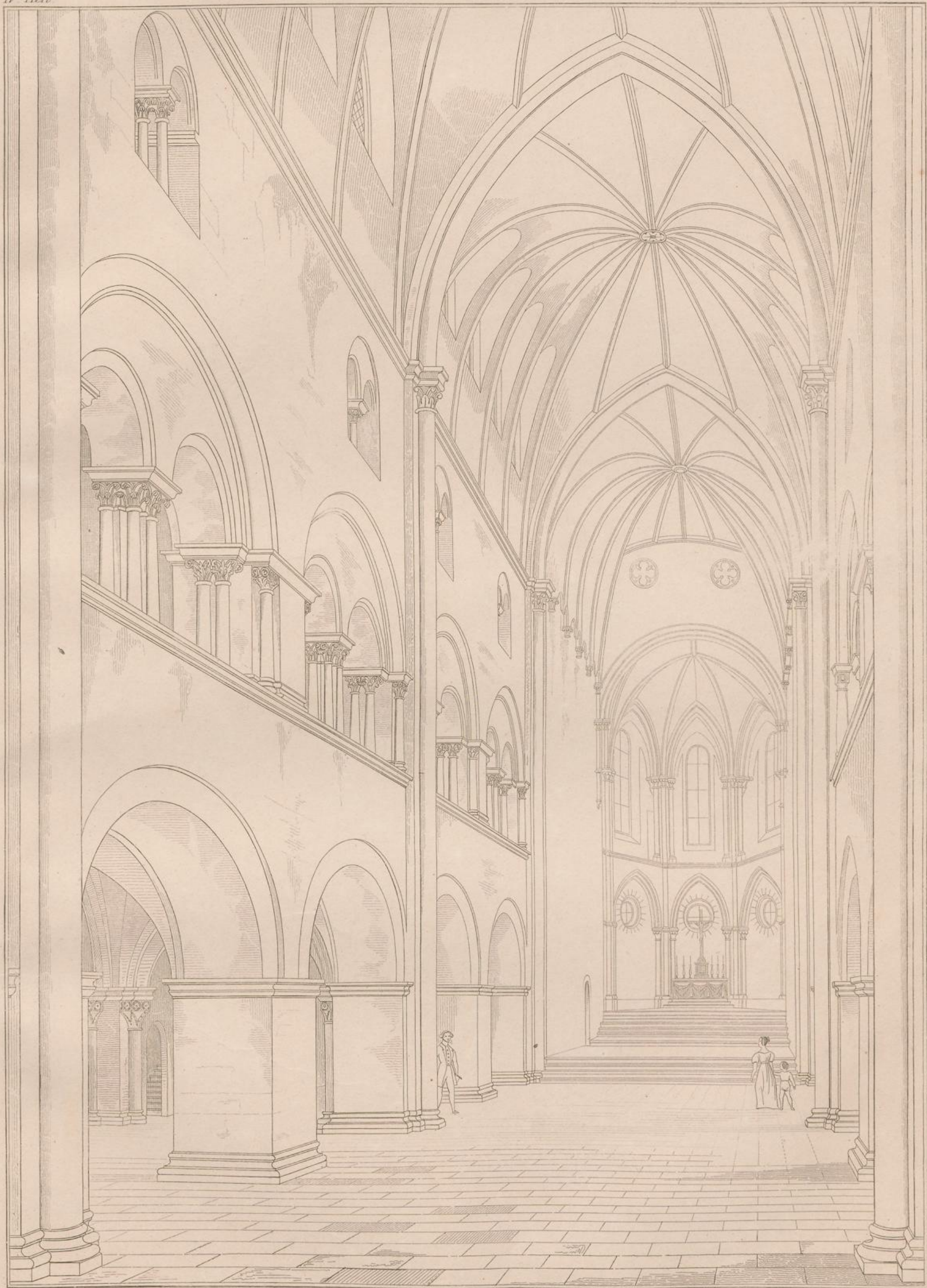
Innere Ansicht der Kirche zu Boppard am Rhein
