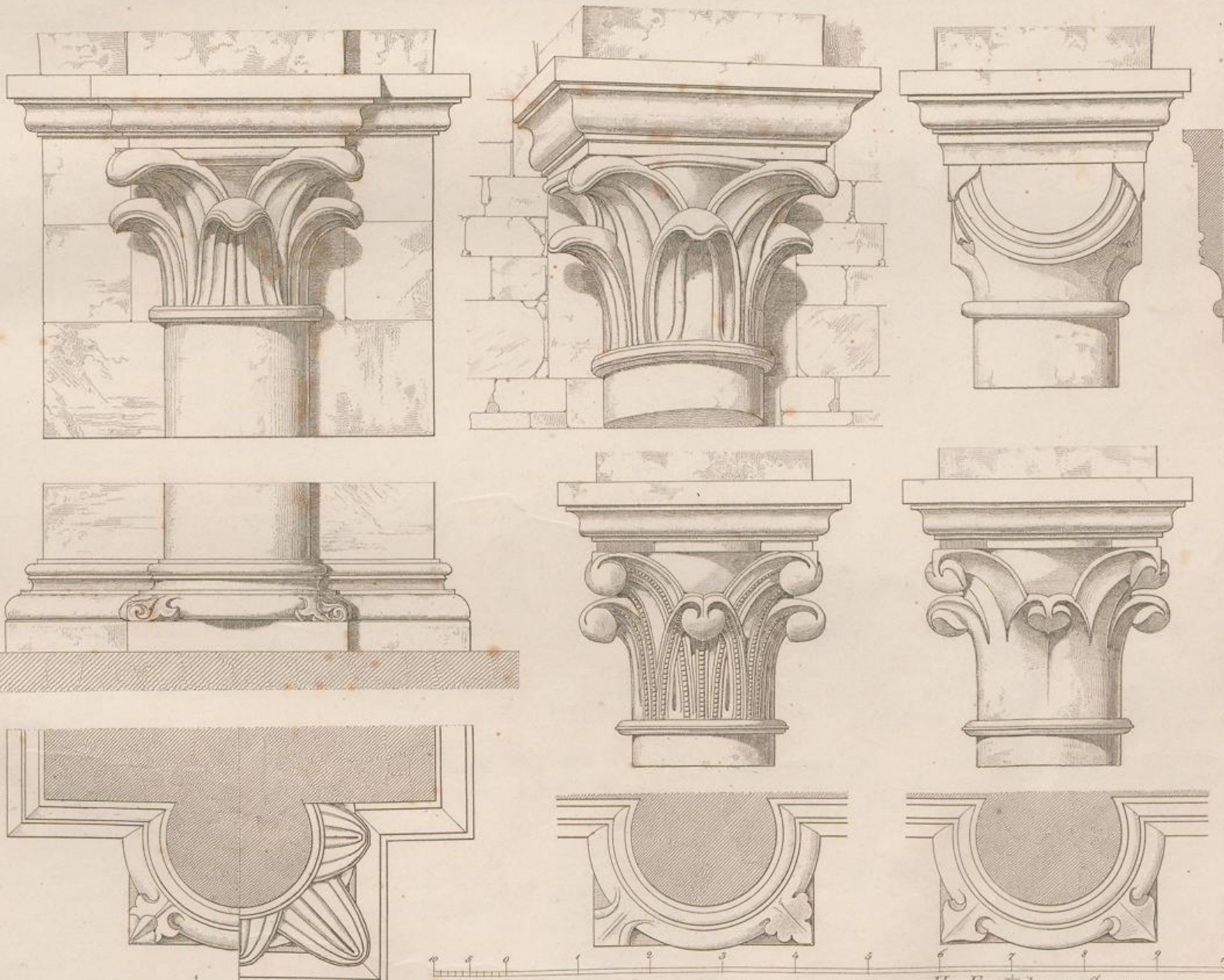
Details der Halbsäulen in den Seitenschiffen
