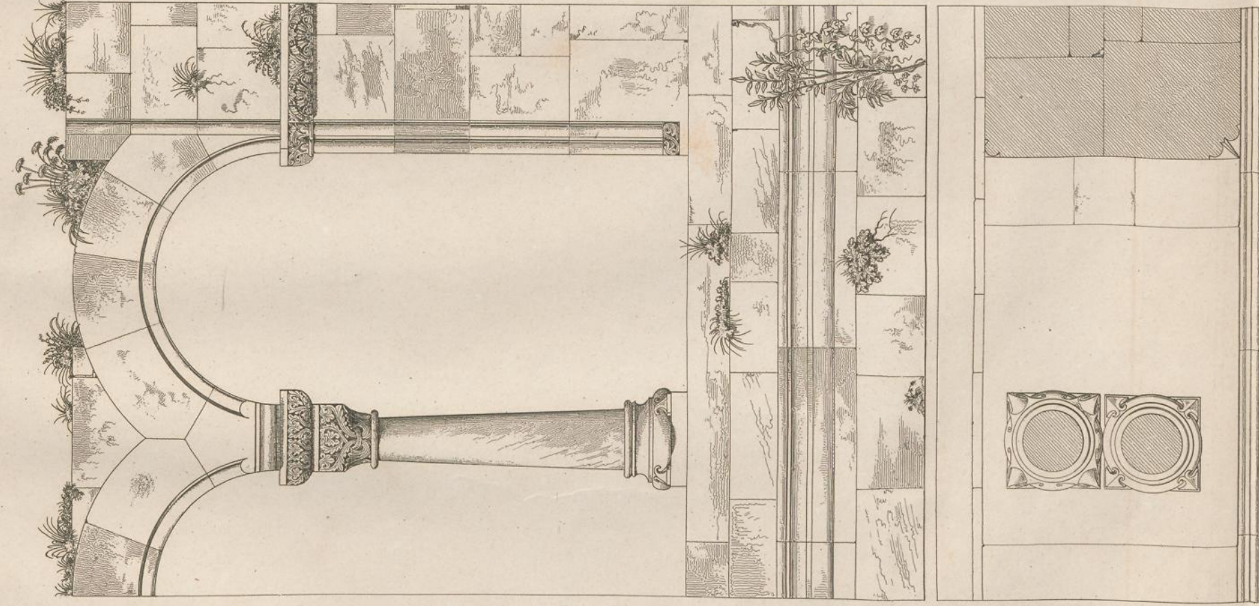
Durchschnitt, Ansicht und Grundriss der Bogenstellungen der vorderen Fassade
