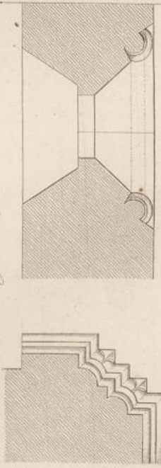
Ansicht und Grundriss der Fenster Details des Portals
