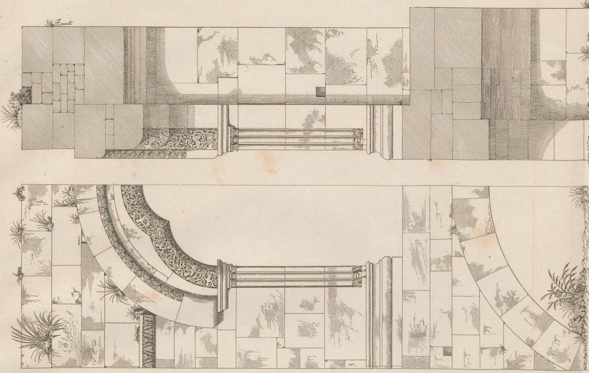
Halbe Ansicht und Durchschnitt des Portals der vorderen Fassade
