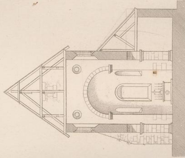
Quer-Durchschnitt
