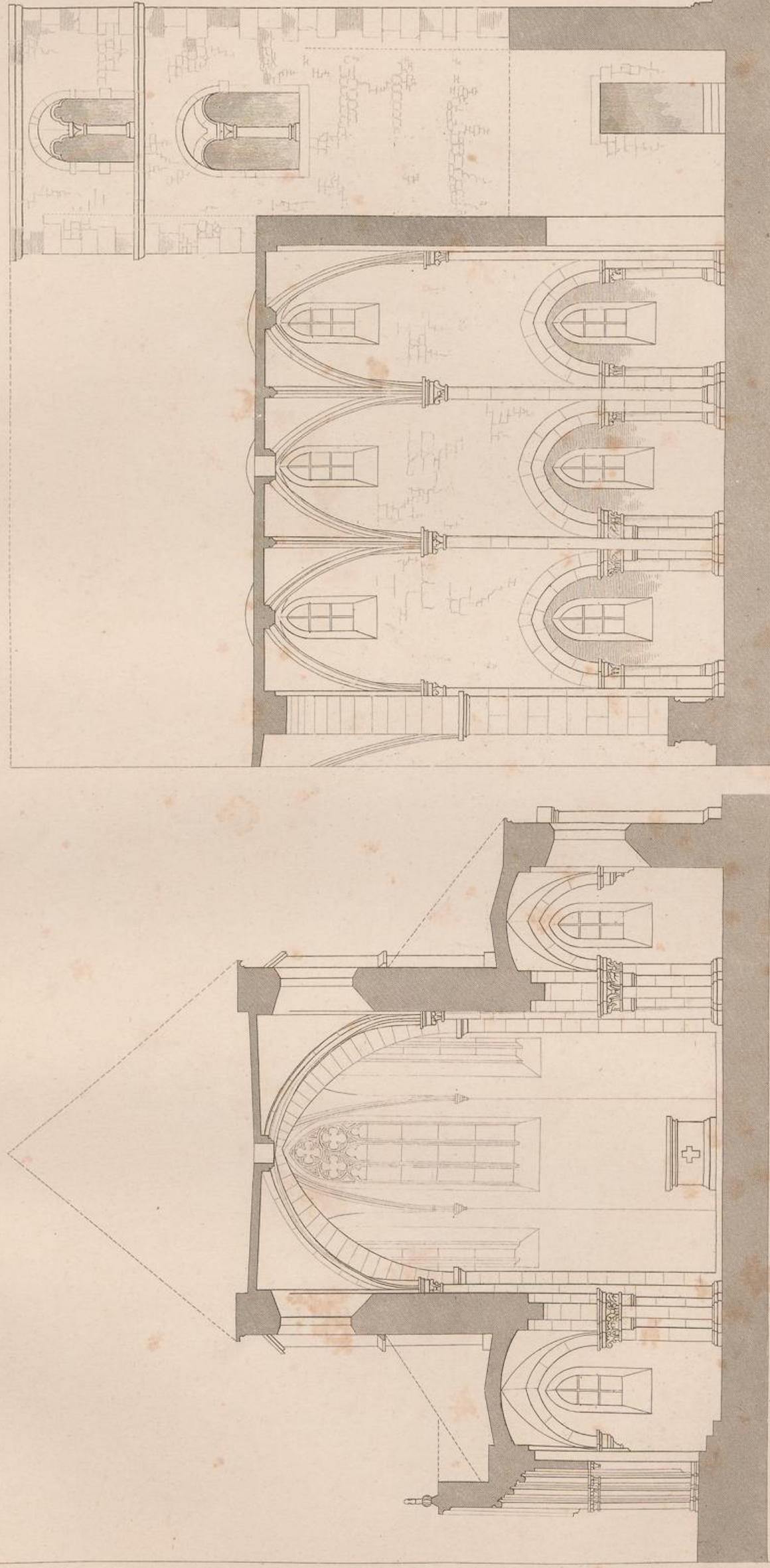
Querdurchschnitt.
