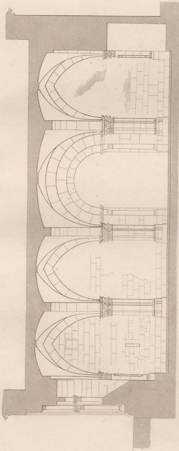
Längenschnitt
