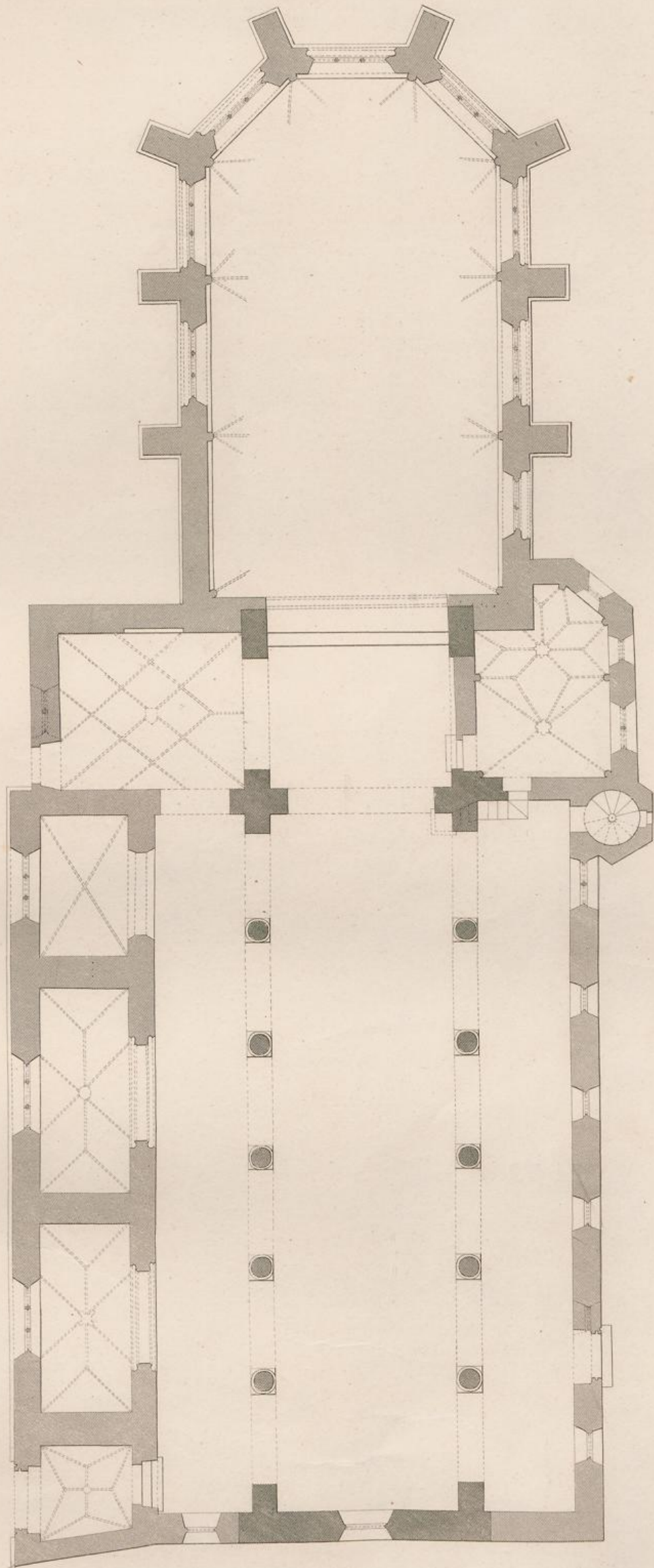
Grundriss der Kirche zu Höchst
