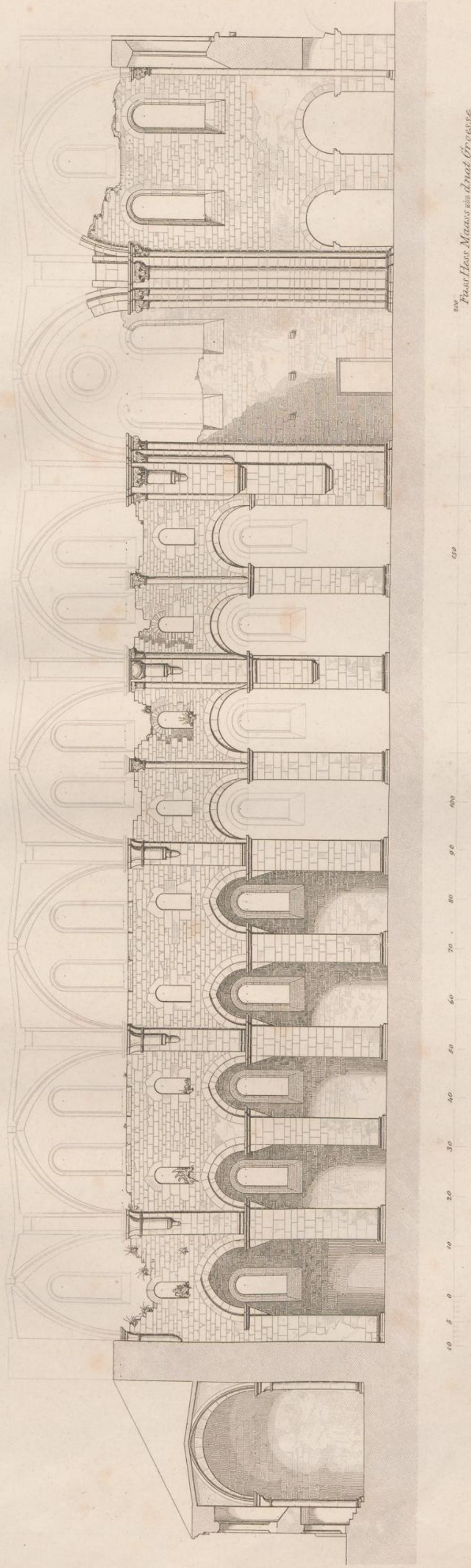
Laengen Durchschnitt
