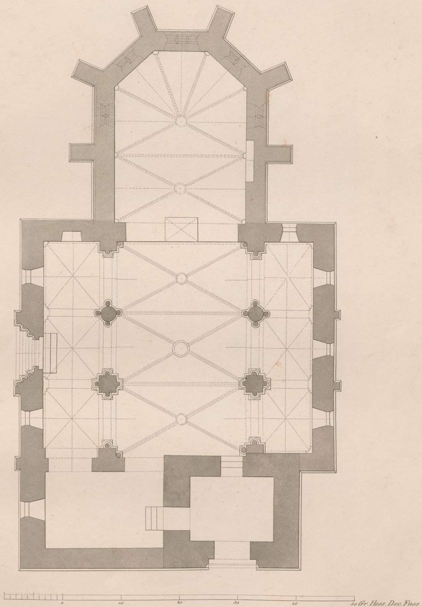
Plan de l'église à Geismülla
