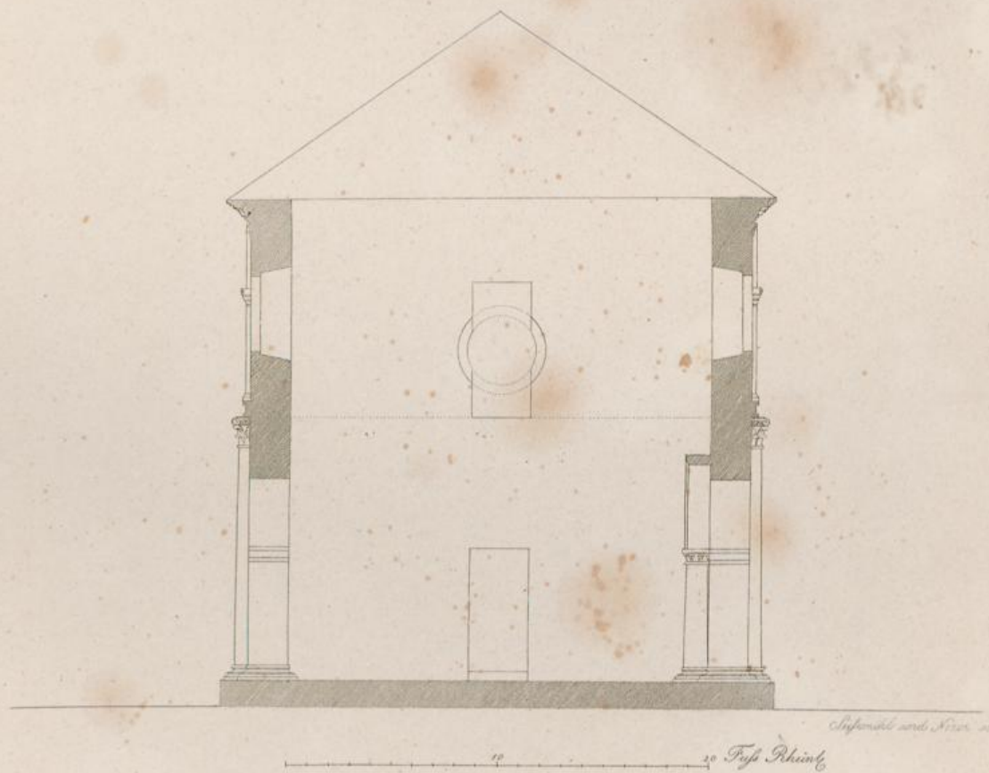
Seiten-Ansicht und Querschnitt der Vorhalle des Klosters Lorsch. Elevation laterale et coupe du vestibule de l'abbaye de Lorsch.
