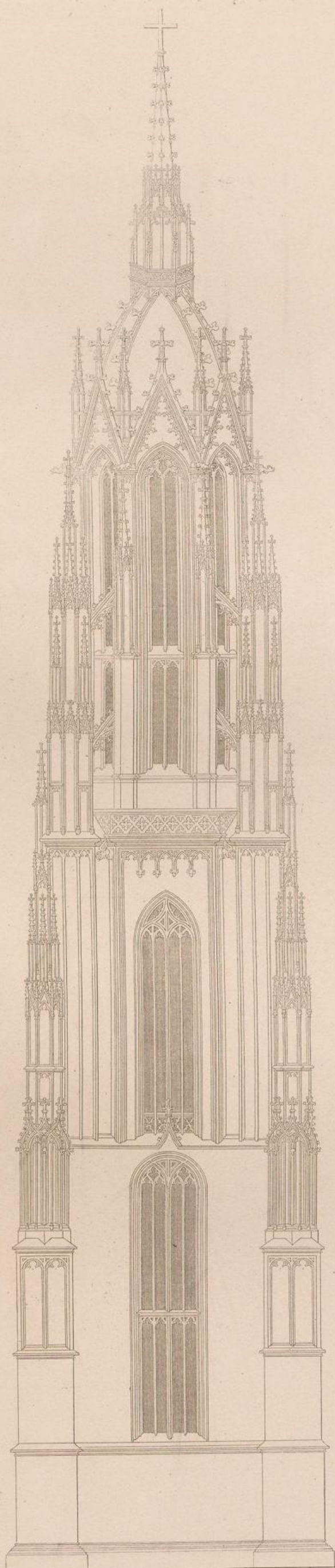
Aufriß des Thurmes der S. Bartholomäus Kirche zu Frankfurt am Main. Elevation du clocher de l'église S. Bartholomay à Francfort sur le Main.
