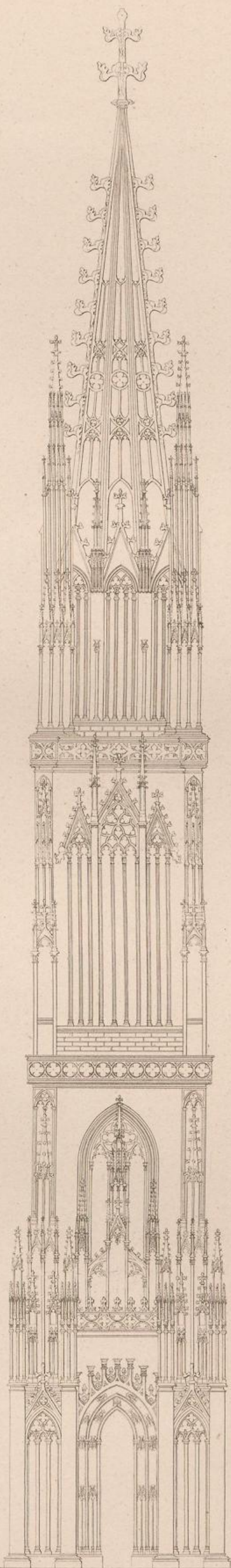
Aufsatz eines Kirchenturmes, nach einer Zeichnung aus dem 14. Jahrhundert, deren Mittheilung man dem Herrn Galleriedirector Becker in Carlsruhe verdankt. Elevation d'un clocher d'après un dessin par parchemin du 14 me siècle.
