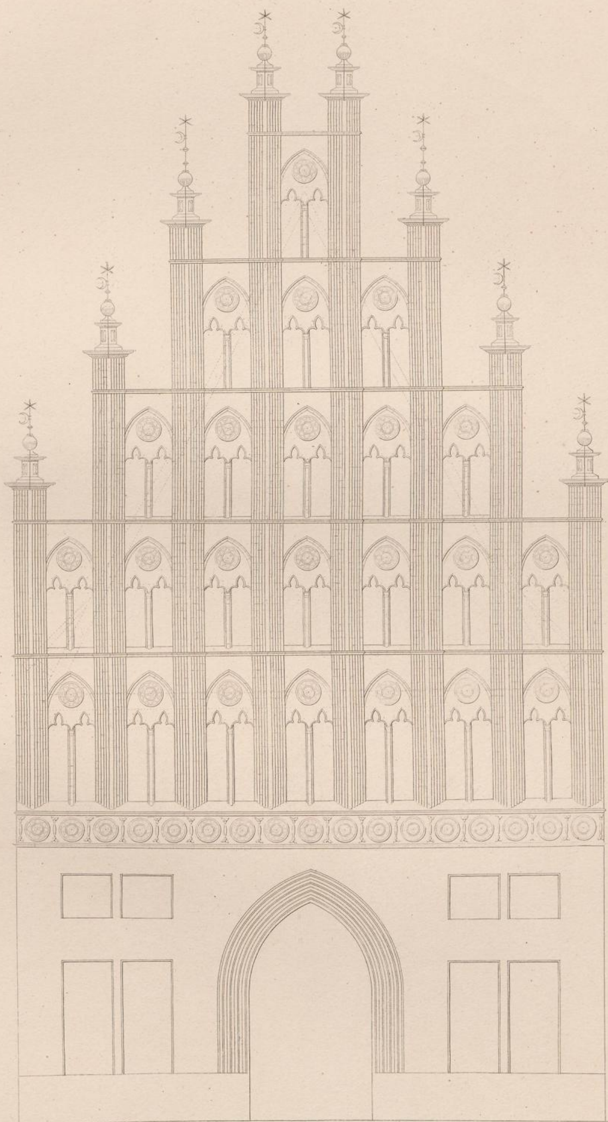
Ansicht eines Hauses zu Hannover in der Knochenhauerstraße. Die Abtheilung der Zeichnung verdankt man dem Herrn Hofbaumeister Witting, d. d. 1811. Façade d'une maison d'Hannovre, rue des bouchers.
