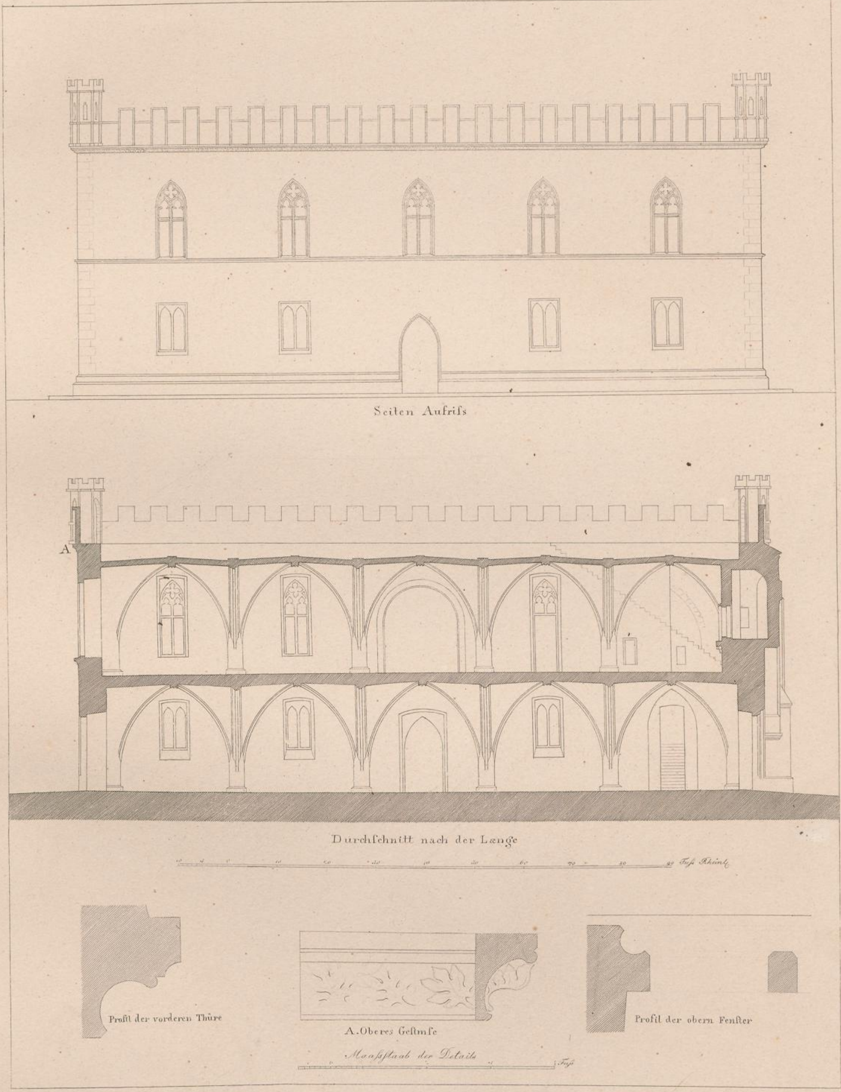
Seitenansicht Durchschnitt und Details des Haupthauses zu Mainz. Façade latérale, coupe et détails de la douane à Mayence.
