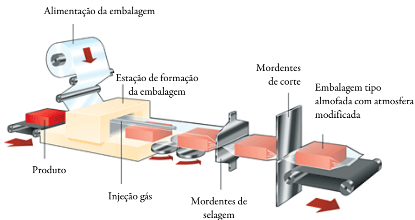
Figura 5.4 - Esquema básico de um equipamento horizontal que forma-enchefe ( http://www.airproducts.com.uk )
