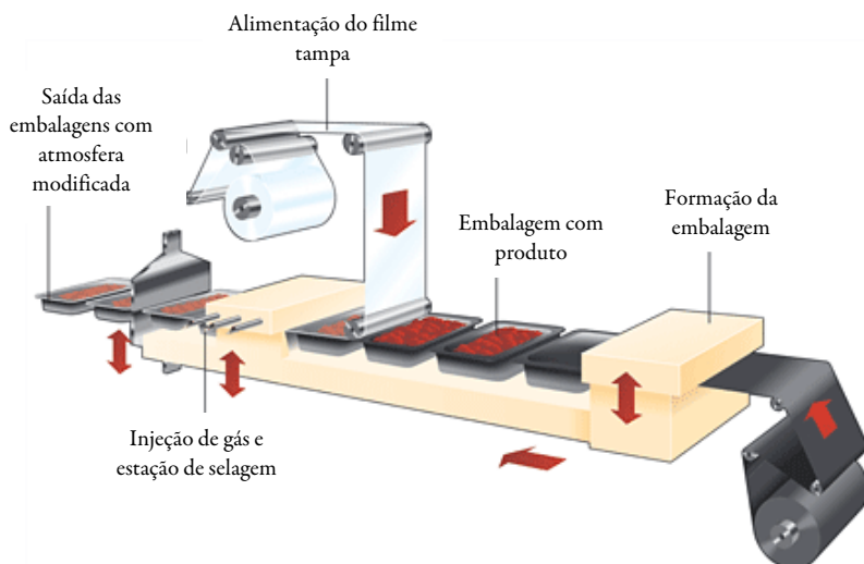
Figura 5.6 - Esquema básico de um equipamento que termoforma-enche-fecha horizontal ( http://www.airproducts.com.uk ).
