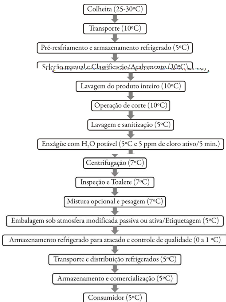
Figura 2.1- Fluxograma geral demonstrando a cadeia produtiva na qual se insere as operações de uma unidade industrial de processamento mínimo de frutas e hortaliças e a temperatura máxima recomendada em cada etapa de processo
