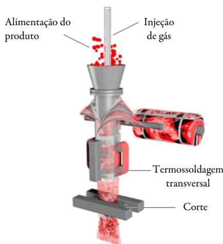
Figura 5.5 - Esquema básico de um equipamento vertical que forma enchefe ( www.ulmapackaging.com/packaging-machines/vertical-vffs )
